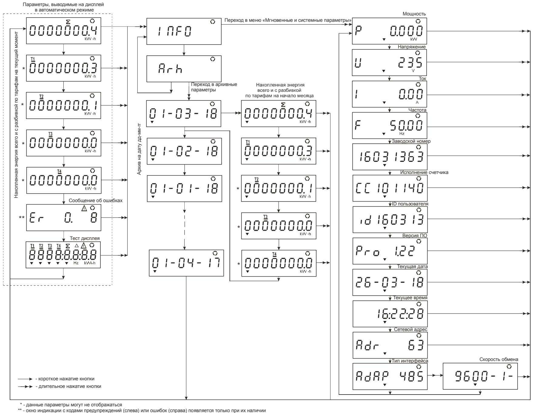
Рисунок 3.2 – Структура вывода информации на дисплей счетчиков «Гран-Электро СС-101-XXXВ»
