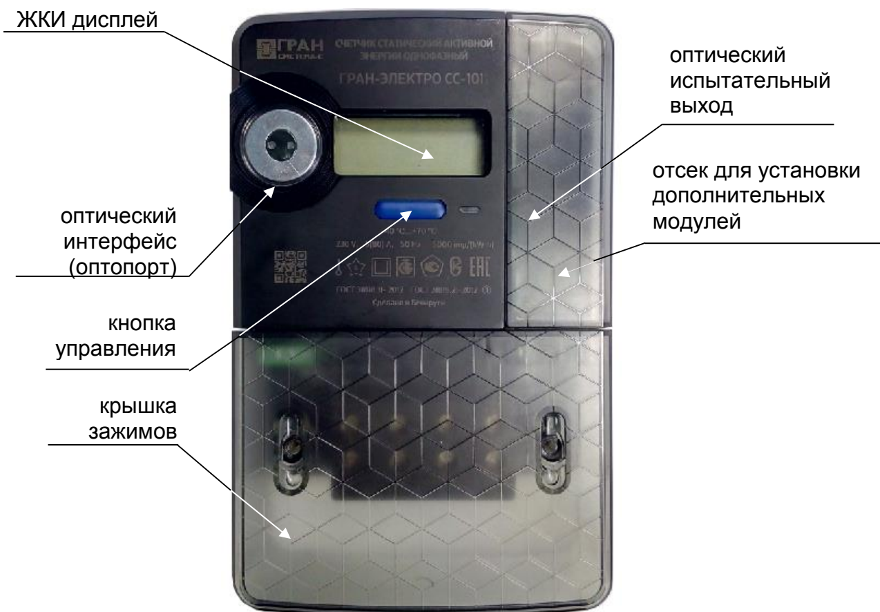
Рисунок 1.4 – Внешний вид счетчиков «Гран-Электро СС-101-XXXВ»
