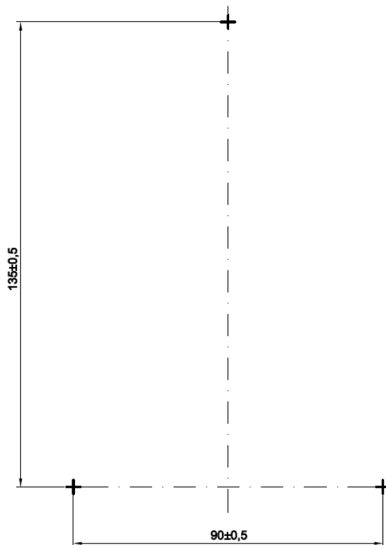
Рисунок А.1 – Габаритные размеры счетчиков «Гран-Электро СС-101-ХХХВ»
