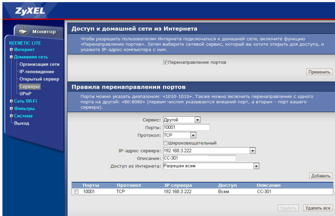
Рисунок Б.3. Пример настройки маршрутизатора ZyXel
